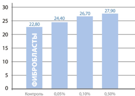
График повышения активности супероксиддисмутазы Активность супероксиддисмутазы была оценена в нескольких концентрациях
